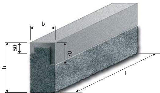
Krawężnik drogowy A
