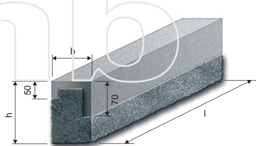
Krawężnik mostowy B
