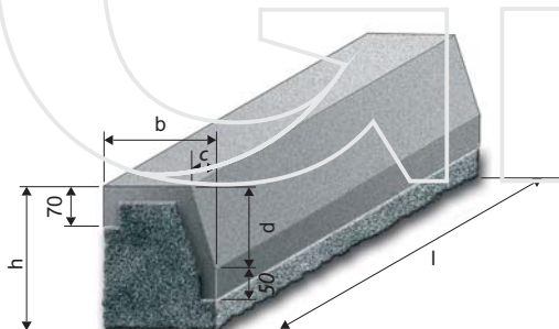
Krawężnik mostowy A
